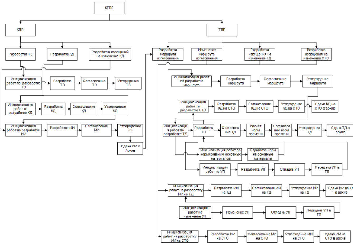
рис. 3. Схема процессов конструкторско-технологической подготовки производства
