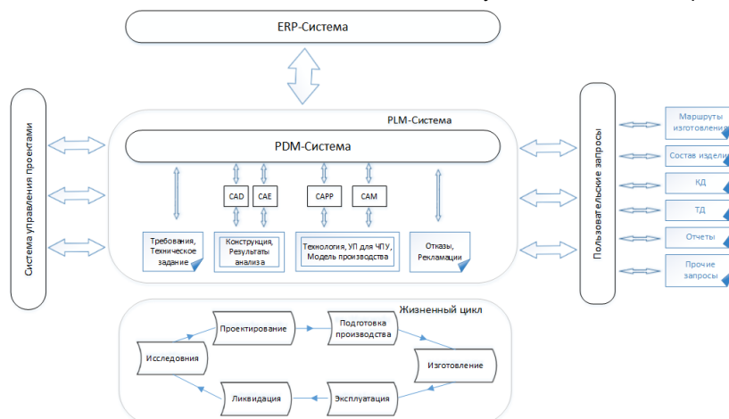
рис. 1. Схема взаимоотношений CAD, CAM, PLM и ERP-систем
